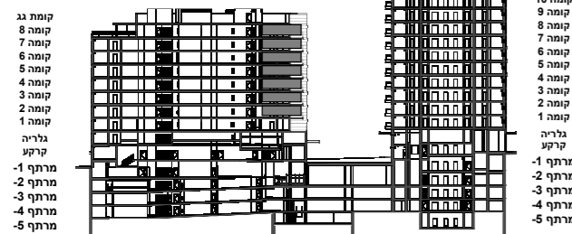
מפתח קומות
