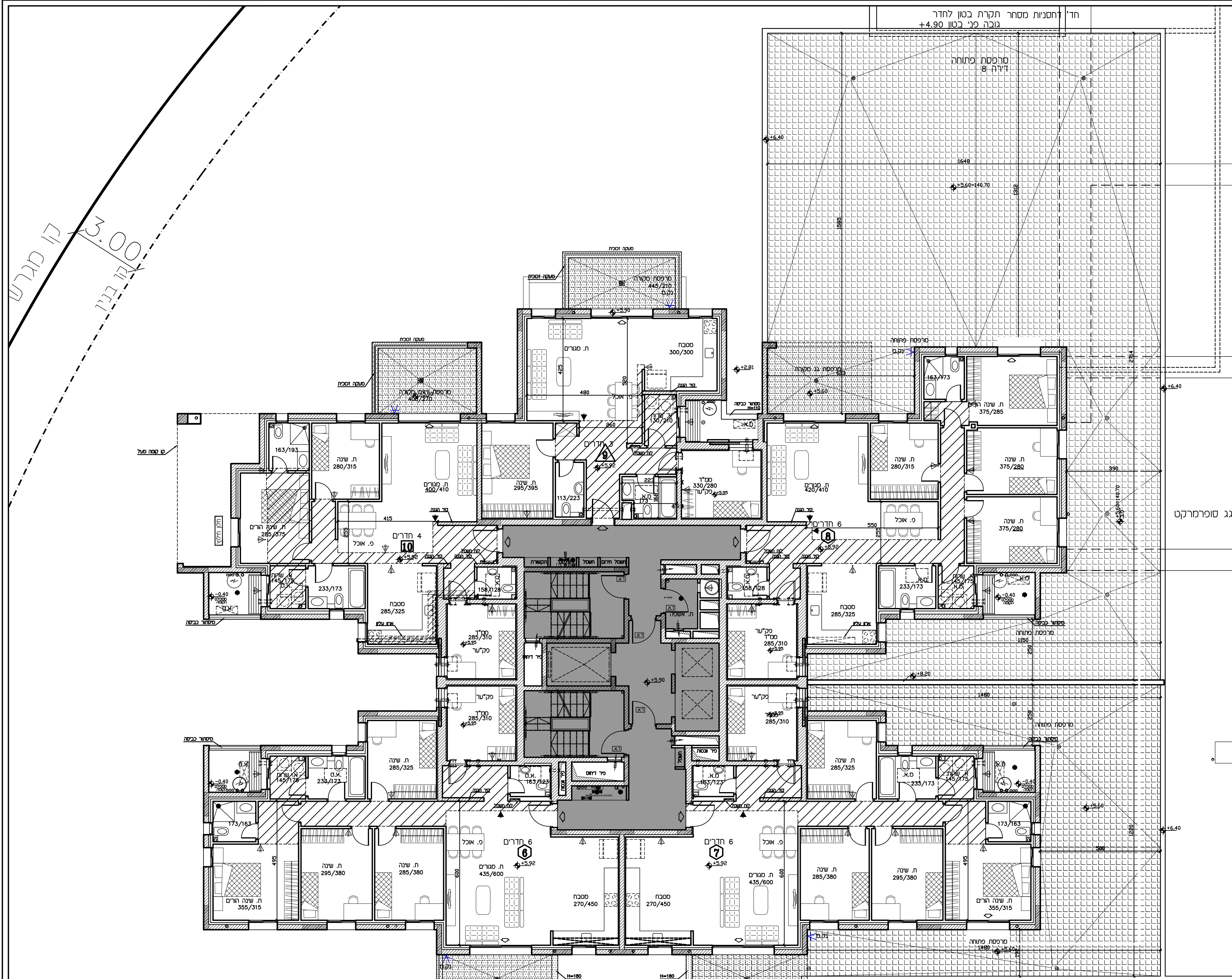
טיפוס E תכנית קומה 2 ק.מ. 1:100
